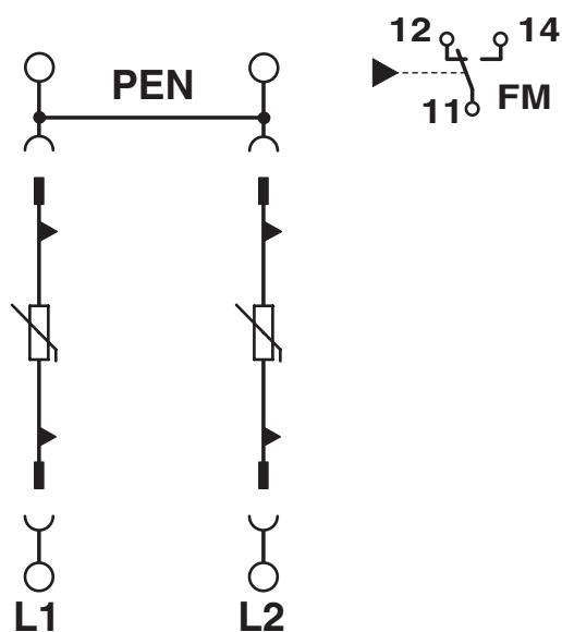
Schemat
