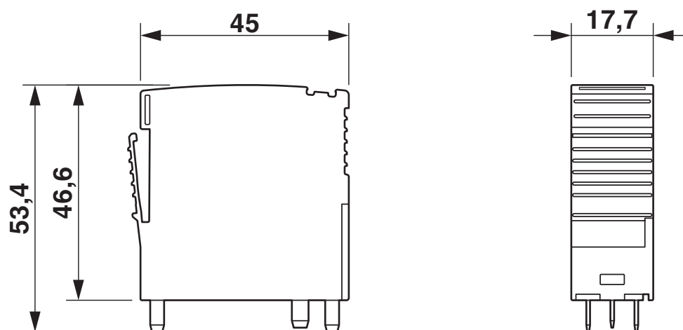
Rysunek wymiarowy
