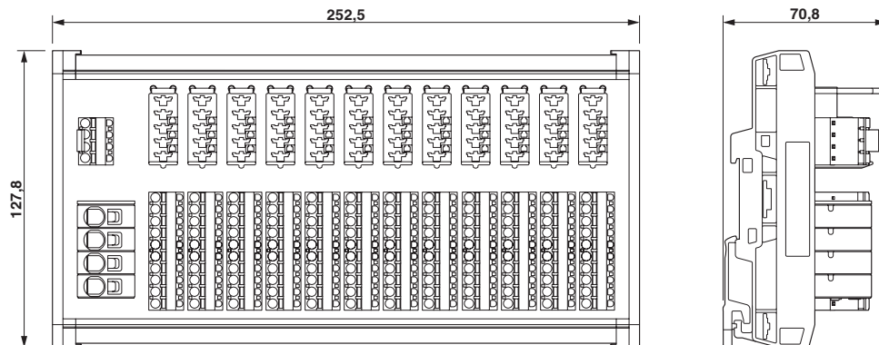
Rysunek wymiarowy
