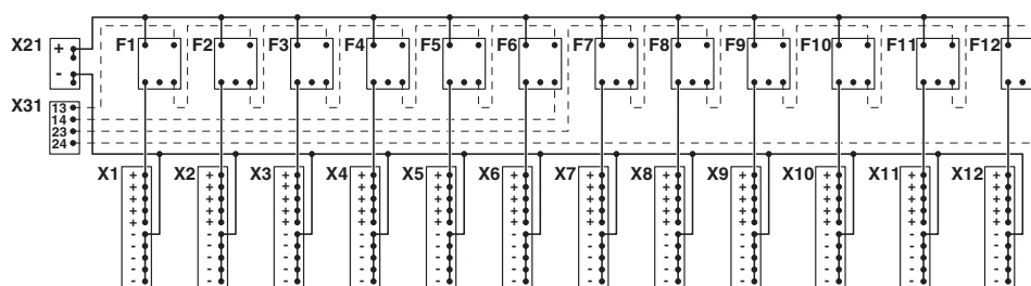
Schemat
