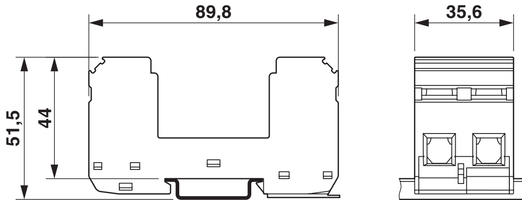
Rysunek wymiarowy
