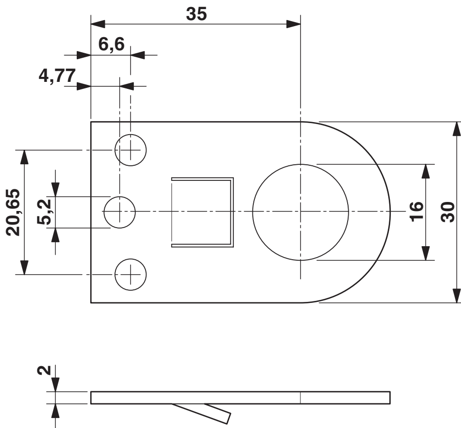
Rysunek wymiarowy
