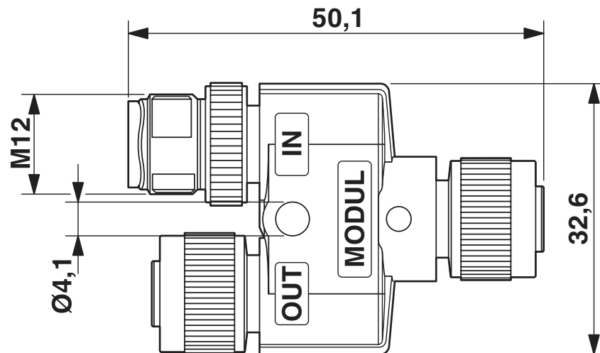
Rysunek wymiarowy
