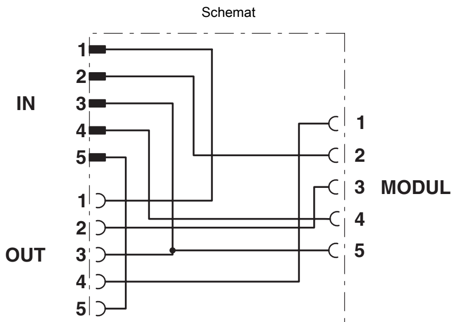
Rysunek schematyczny
