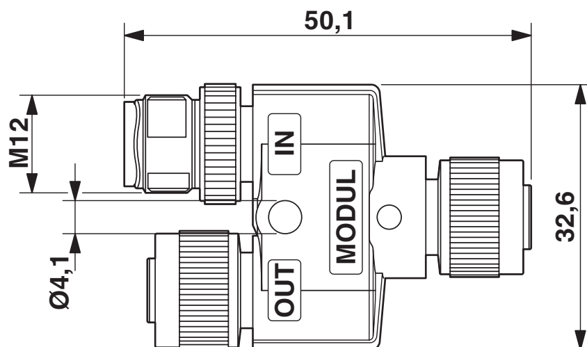
Rysunek wymiarowy
