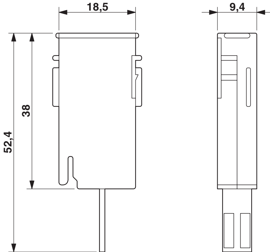
Rysunek wymiarowy
