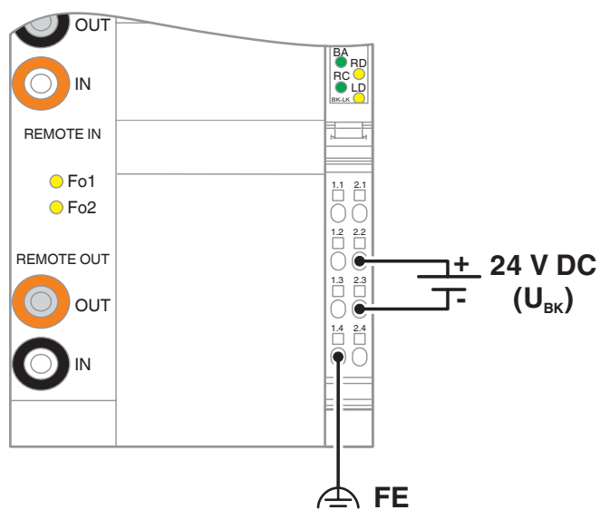
rysunek złączy
