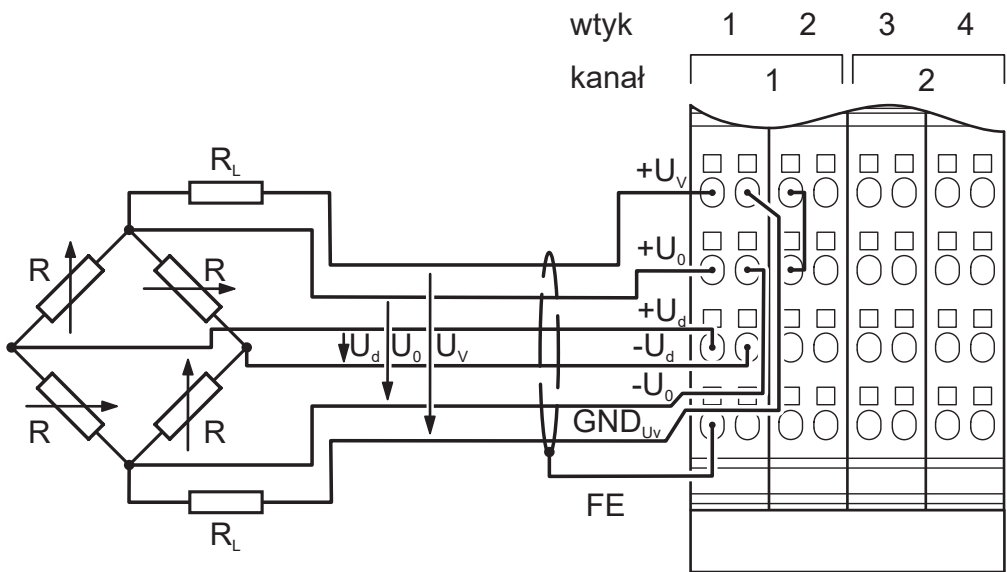
rysunek złączy
