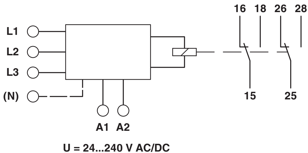
Schemat blokowy
