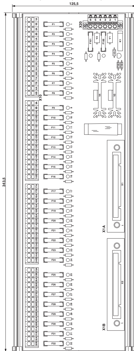
Rysunek wymiarowy
