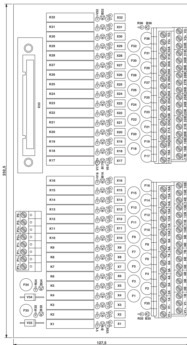
Rysunek wymiarowy
