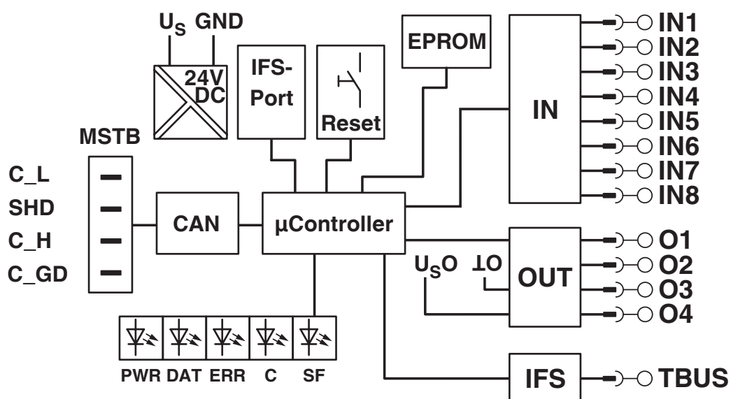
Schemat blokowy
