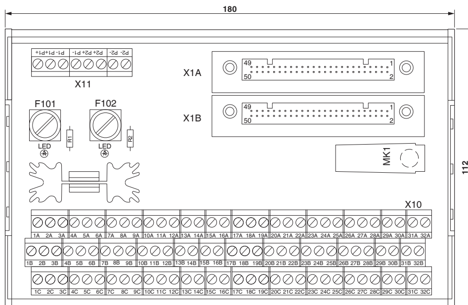
Rysunek wymiarowy
