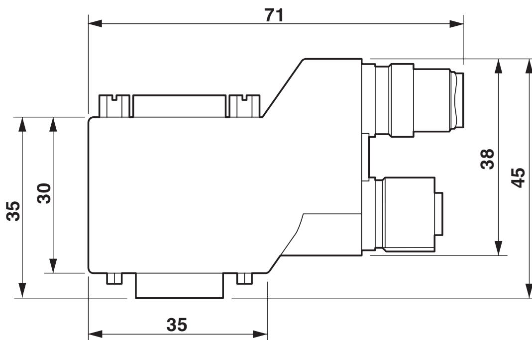
Rysunek wymiarowy SUBCON-PLUS...90...M12, wersja krótka 90°
