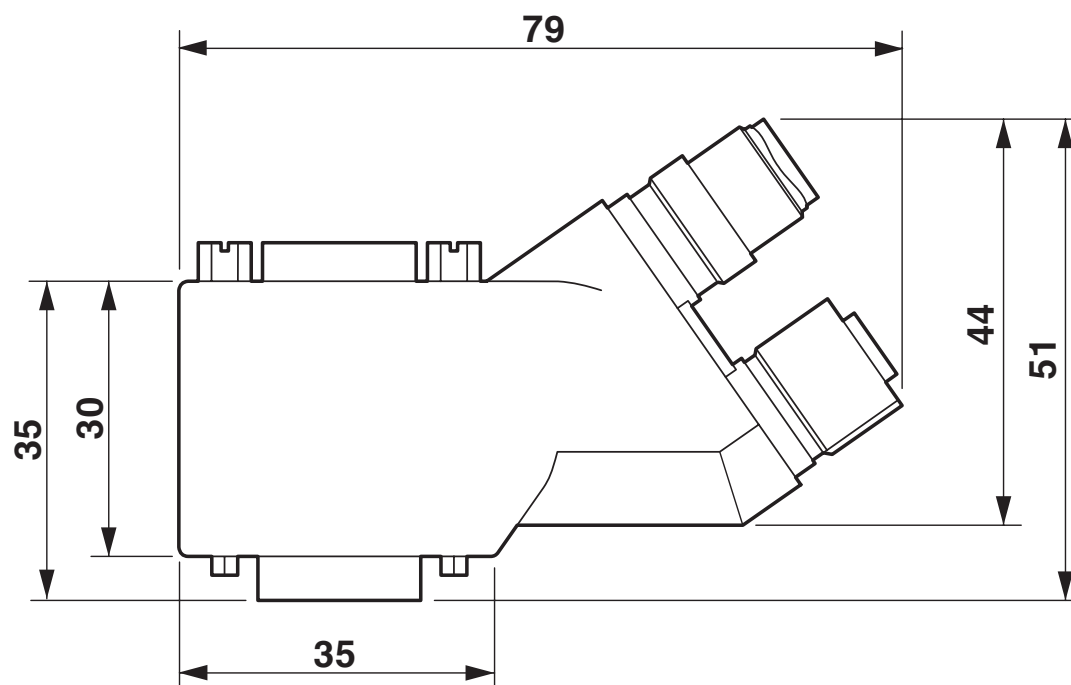
Rysunek wymiarowy SUBCON-PLUS..35...M12, wersja 35°
