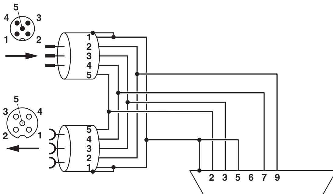
Schemat funkcjonalny SUBCON-PLUS-CAN/...M12
