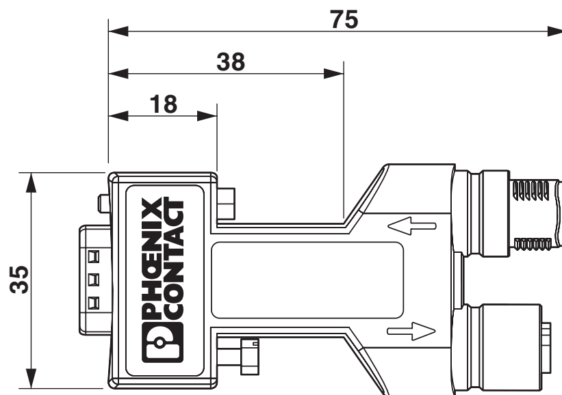
Rysunek z wymiarami SUBCON-PLUS...AX...M12, wersja osiowa (180°)
