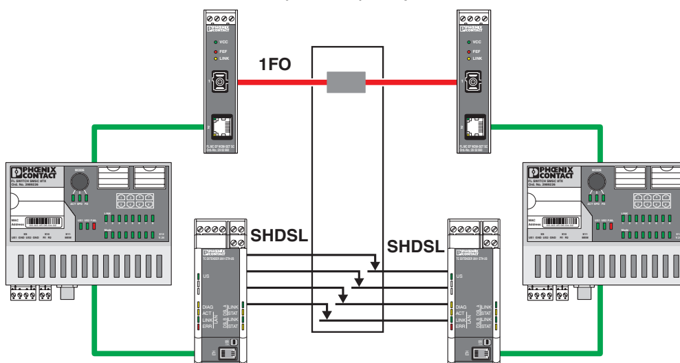
Redundantna komunikacja za pośrednictwem pierścienia ślizgowego
