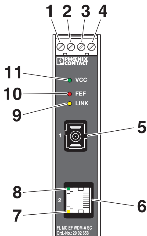
Rysunek schematyczny
