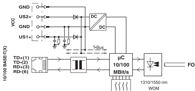
Schemat blokowy
