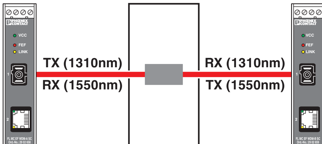
Komunikacja za pośrednictwem pierścienia ślizgowego
