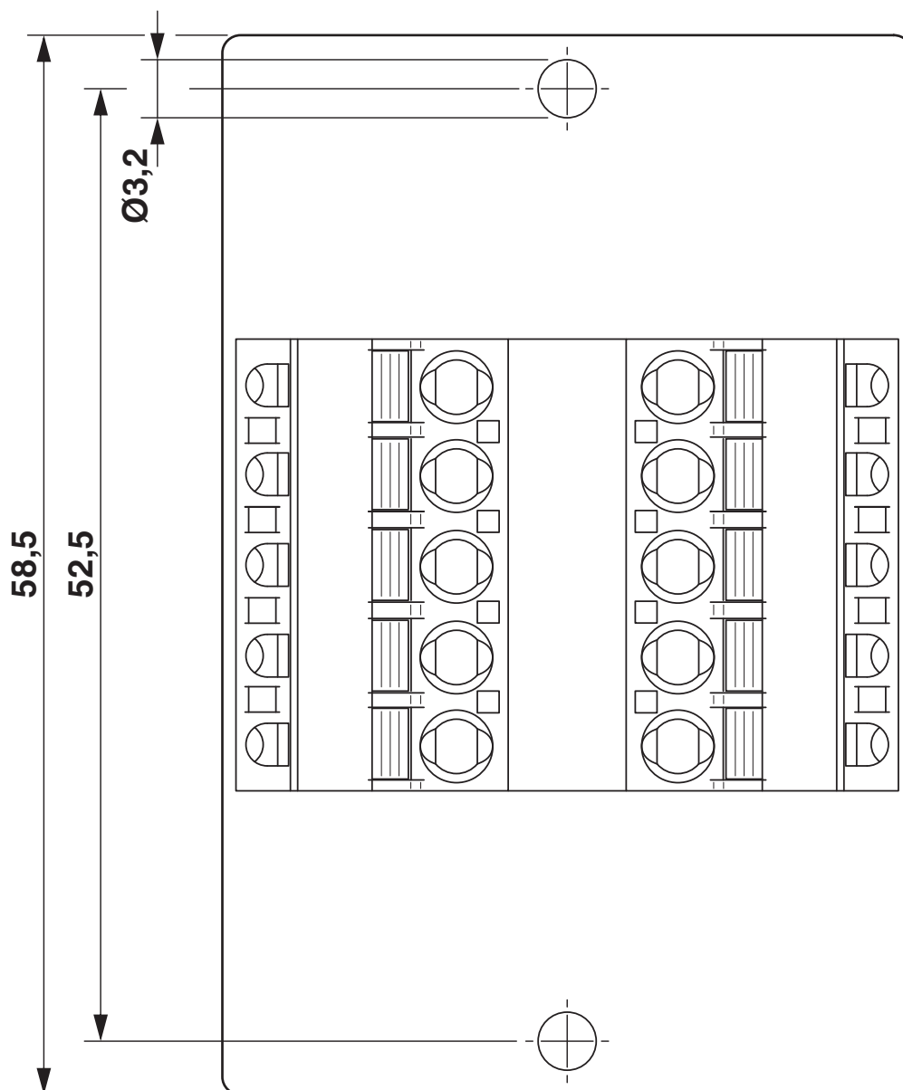
Rysunek wymiarowy
