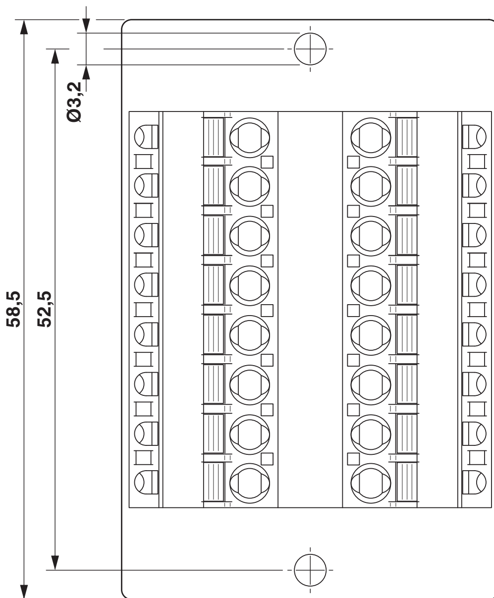
Rysunek wymiarowy
