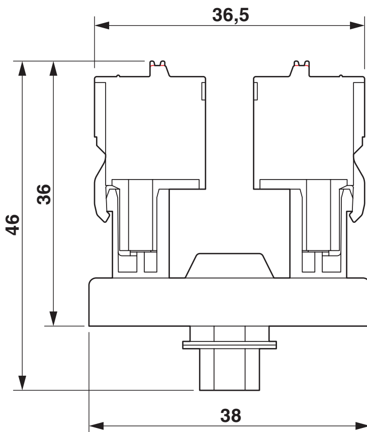
Rysunek wymiarowy
