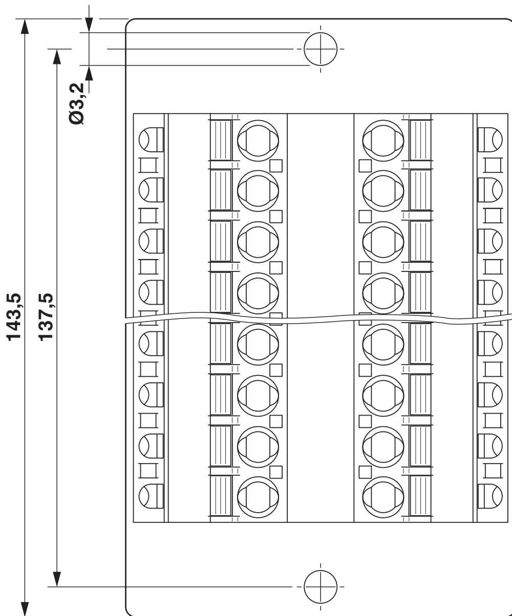
Rysunek wymiarowy
