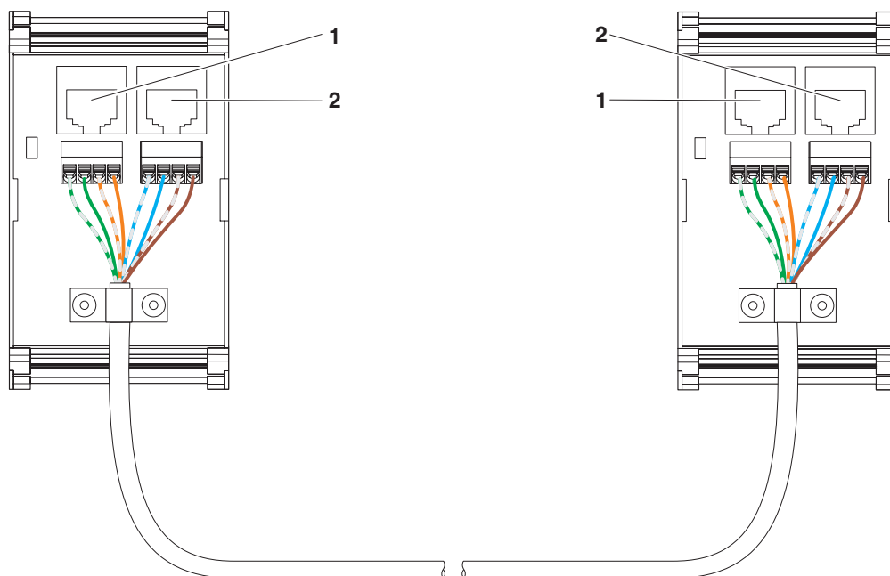
rysunek złączy
