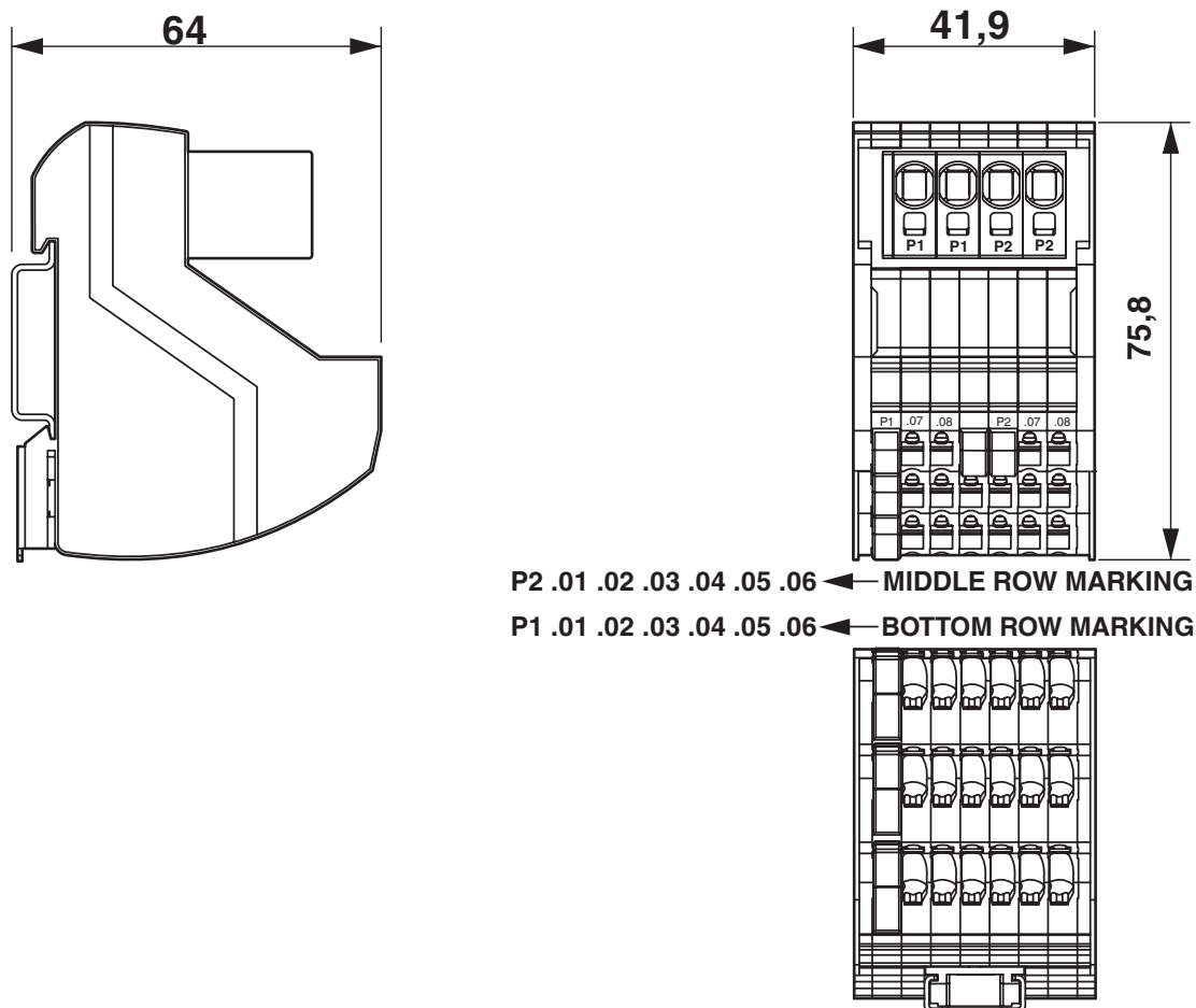
Rysunek wymiarowy
