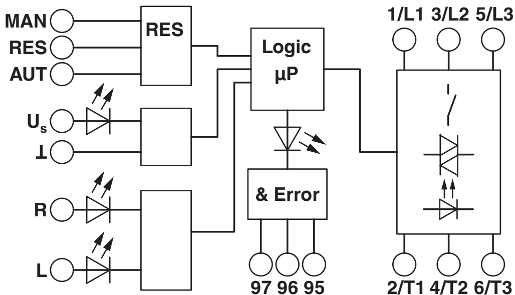
Schemat blokowy
