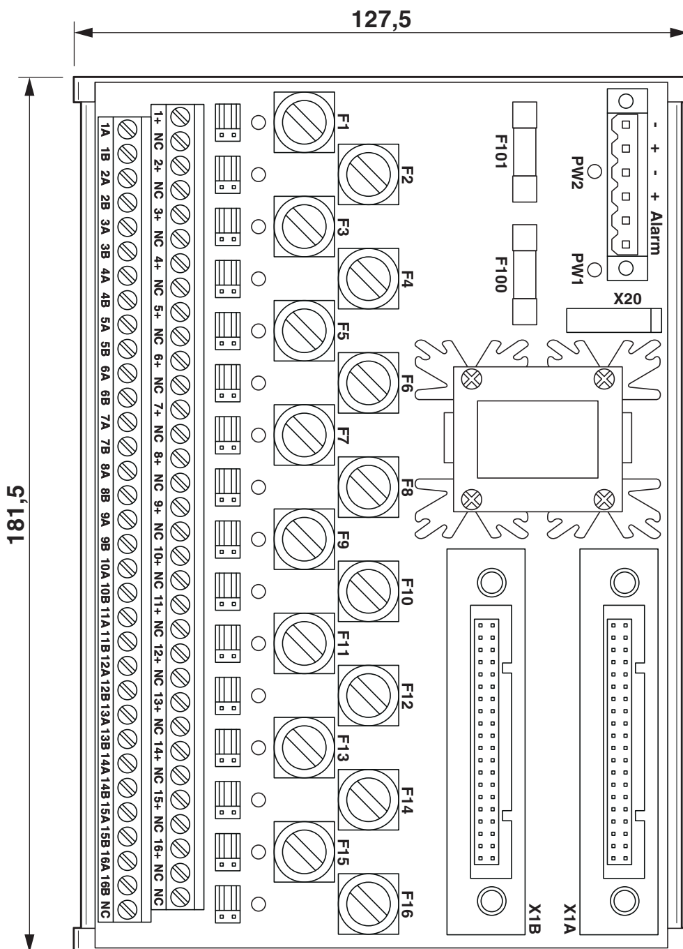
Rysunek wymiarowy
