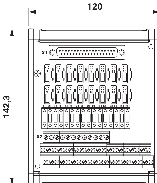
Rysunek wymiarowy
