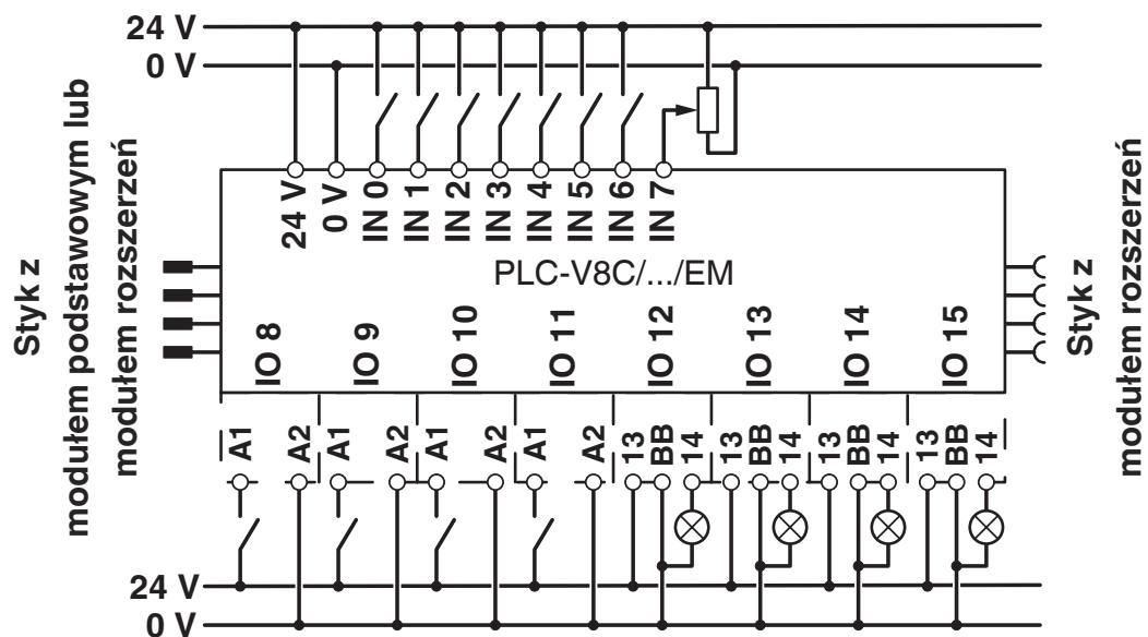
rysunek złączy
