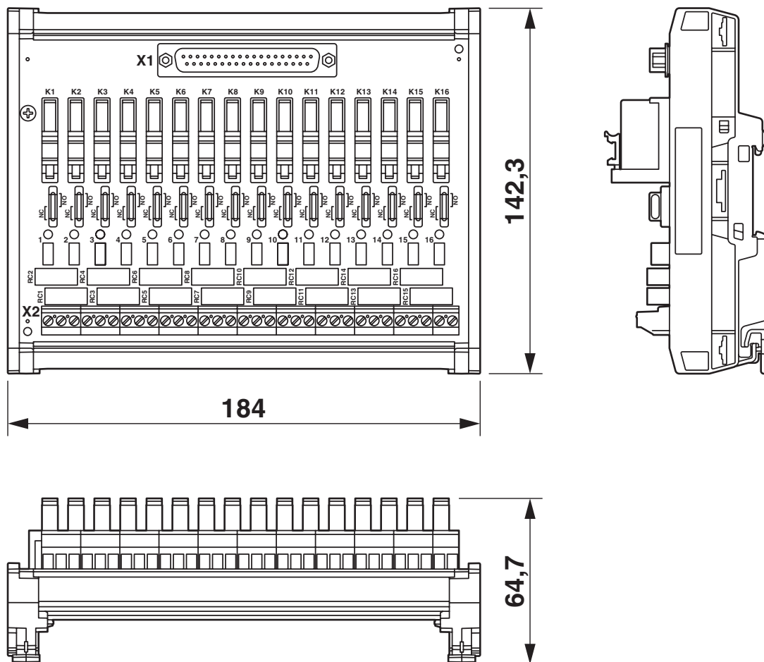
Rysunek wymiarowy
