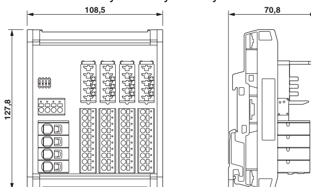
Rysunek wymiarowy
