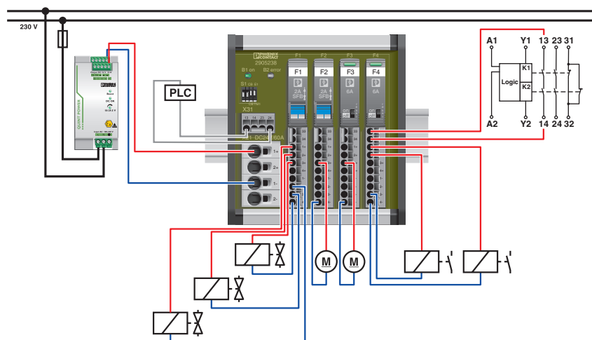
rysunek aplikacji
