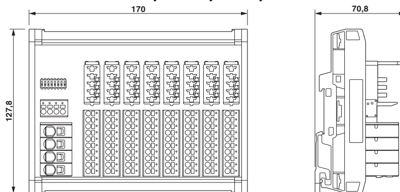
Rysunek wymiarowy
