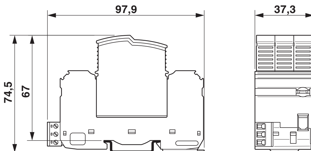
Rysunek wymiarowy
