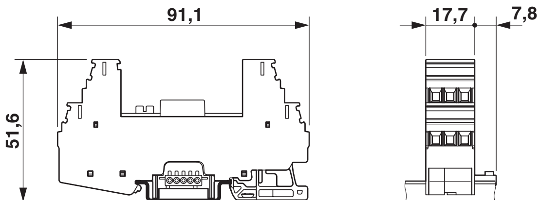
Rysunek wymiarowy
