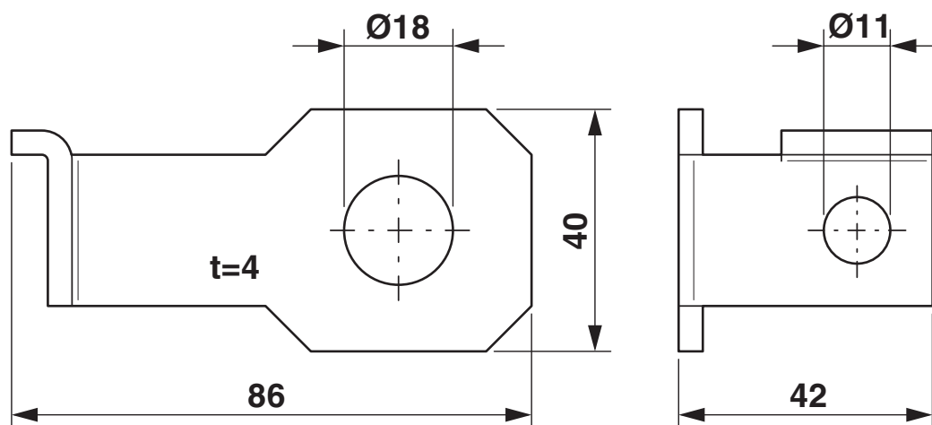
Rysunek wymiarowy
