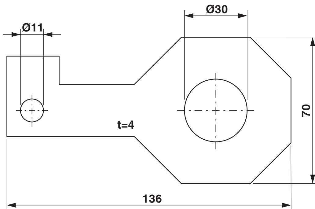
Rysunek wymiarowy
