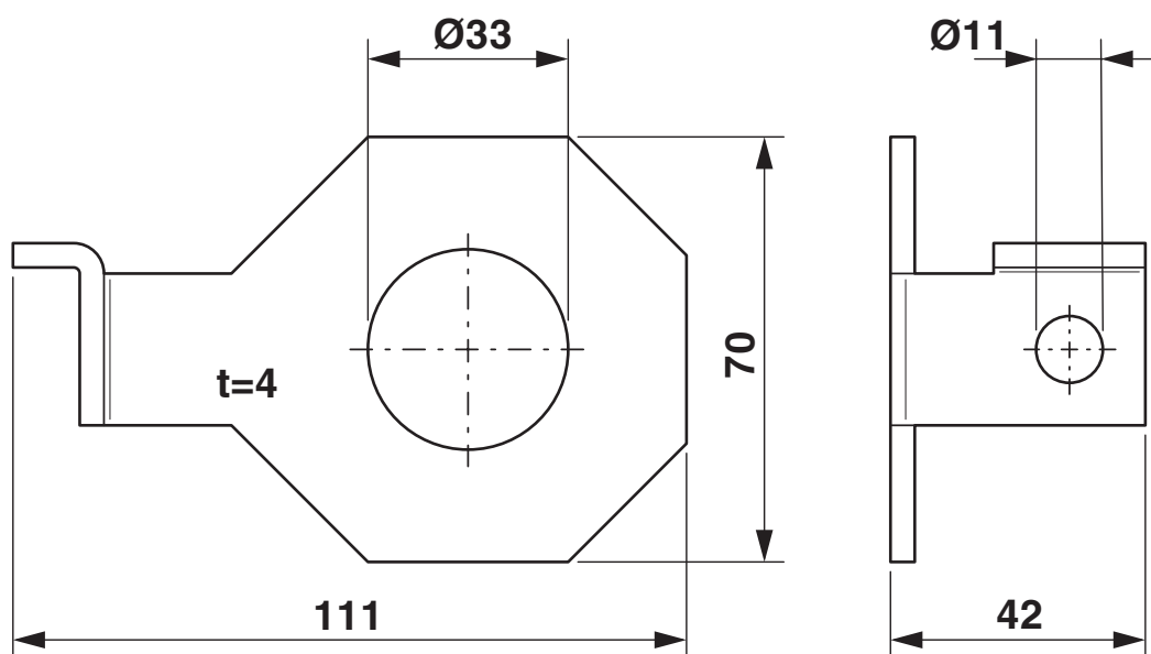
Rysunek wymiarowy
