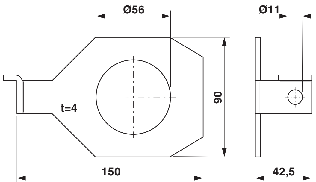
Rysunek wymiarowy
