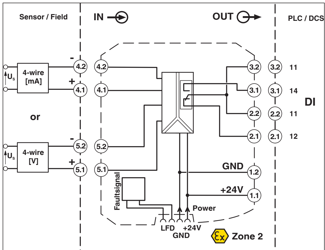
Schemat blokowy
