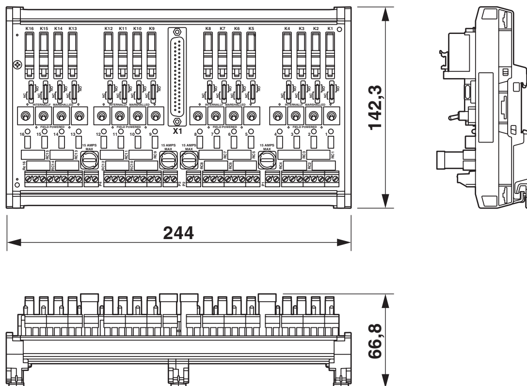
Rysunek wymiarowy
