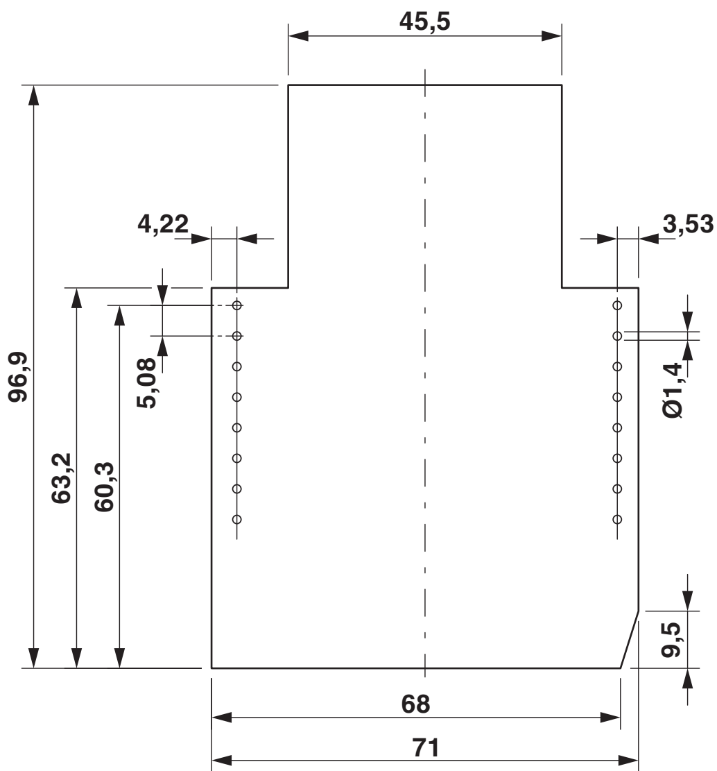
Rysunek wymiarowy
