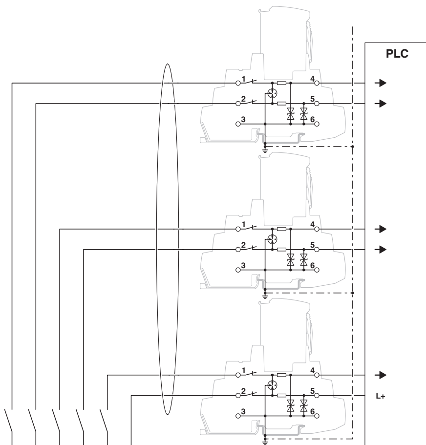
rysunek aplikacji
