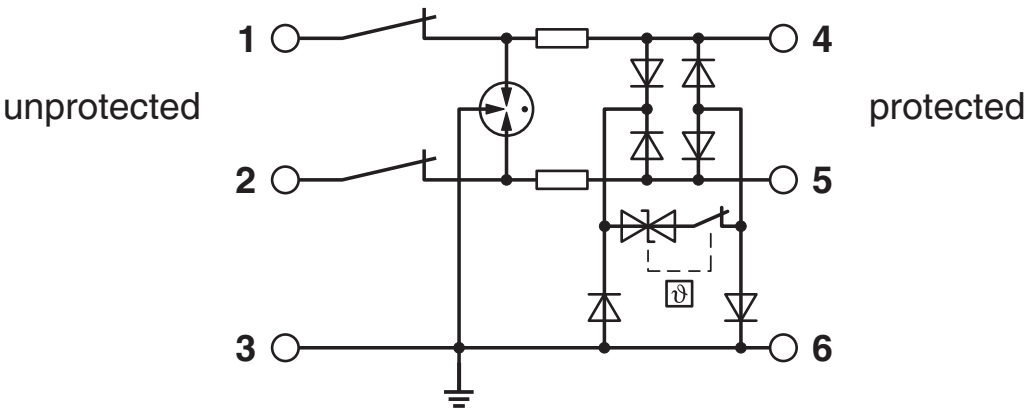
Schemat
