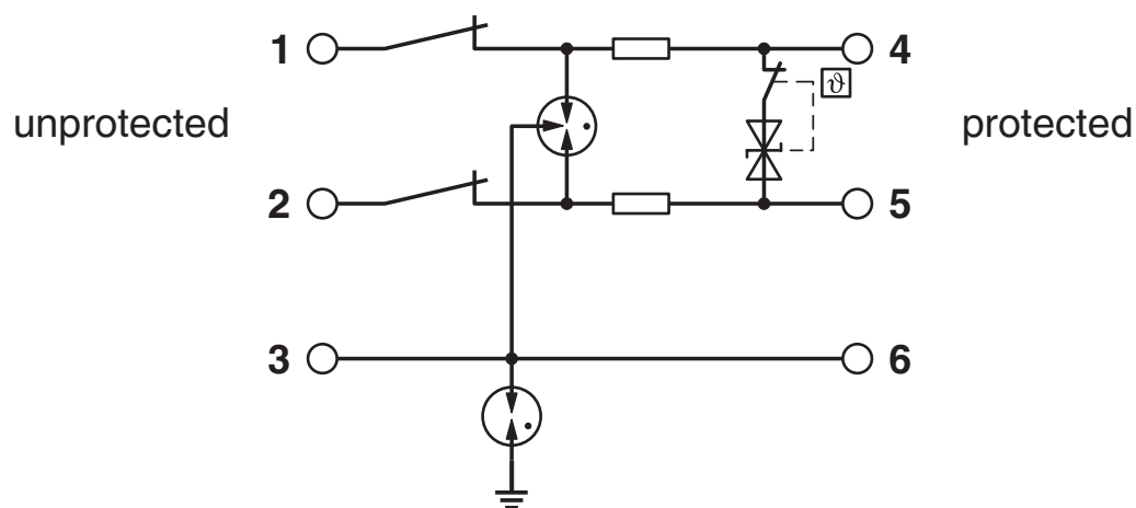
Schemat
