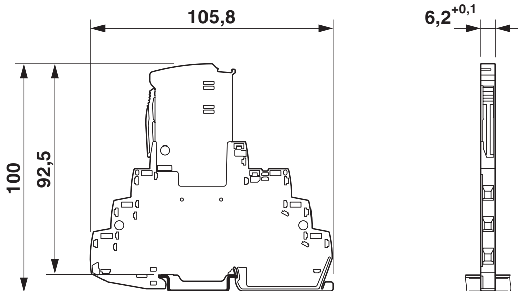
Schemat
