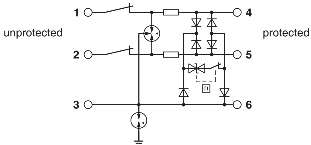
Schemat
