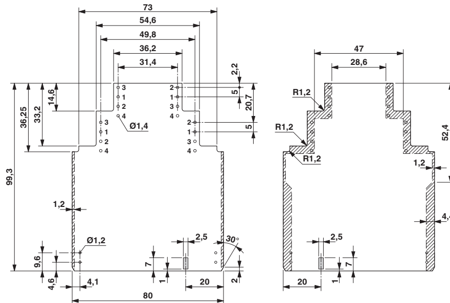
Rysunek wymiarowy
