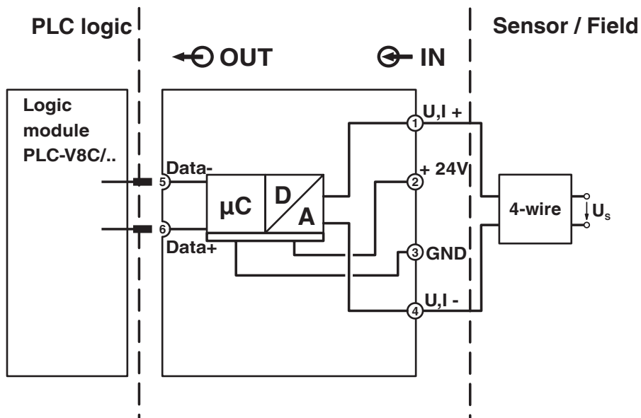
Schemat blokowy
