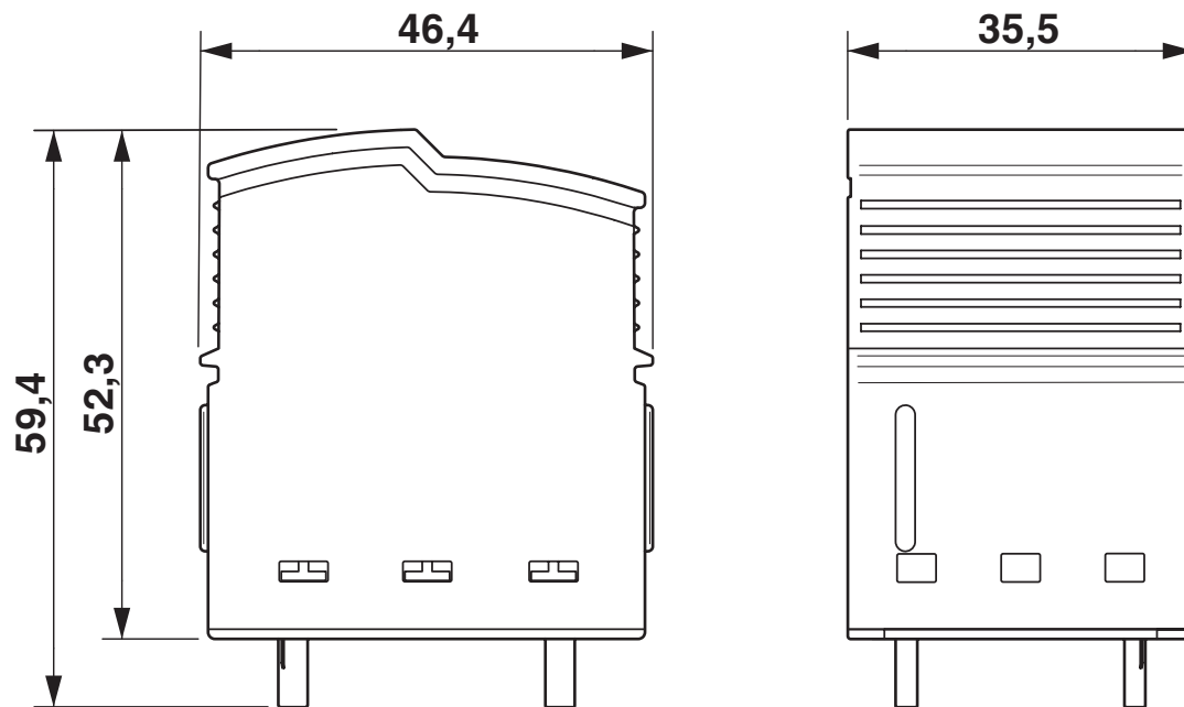
Rysunek wymiarowy
