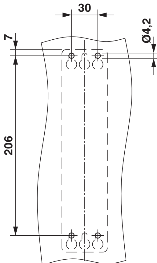
Otworowanie/geometria płytek lutowniczych
