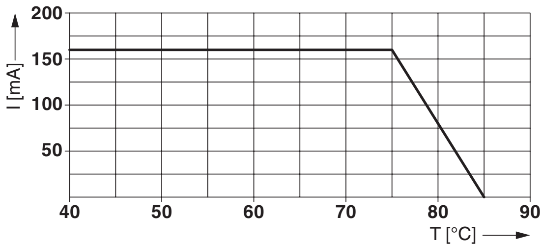
Wykres obniżenia parametrów znamionowych przy 55,2 V DC
