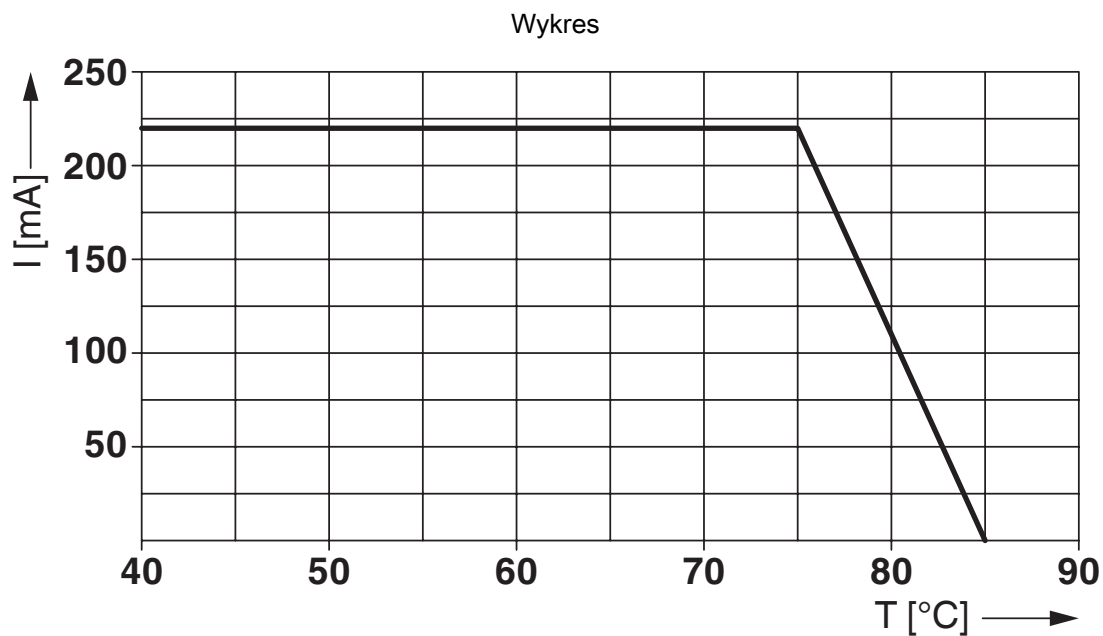
Wykres obniżenia parametrów znamionowych przy 55,2 V DC
